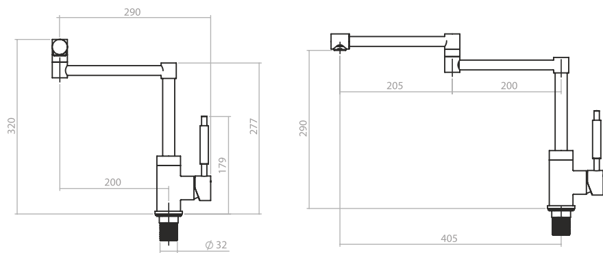
4440 Misturador Monocomando Cozinha Mesa Mixer Kitchen Single Lever Mixer Mezclador Monocomando De Cocina Mixer Código: 6265
