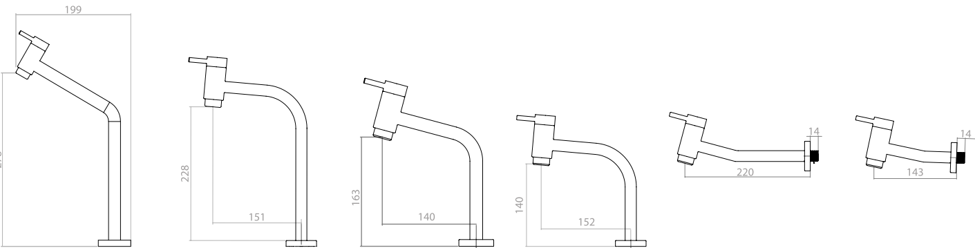
3020 Torneira Parede Slim Wall-mounted Faucet Slim Grifo De Pared Slim Código Acab. C61: 3230 Código Acab. C71: 4717 3000 Torneira Jardim | Tanque Parede com Bico Metal Slim Laundry/tank Faucet Slim With a Nozzle Connector Metal Grifo De Jardim / Tanque Slim Con Pico De Metal Código Acab. C61: 4700 Código Acab. C71: 4721 3801 Ducha Higiênica Slim Hygienic Shower Slim Ducha Higiênica Slim Código Acab. C61: 4701 Código Acab. C71: 4722
