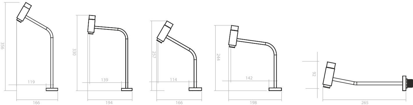
4130 Torneira Lavatório Mesa Slim Platz Bench-top Washbasin Faucet Slim Platz Line Grifo De Lavabo De Mesa Linea Slim Platz Código: 5495
