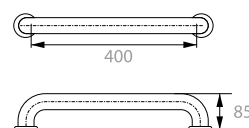
2340 Barra de Apoio 40cm 1 1/4" Bath Grab Bar 40cm 1 1/4" Barra de Apoyo 40cm 1 1/4" Código: 3319
