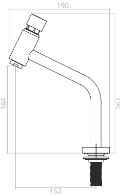
5040 Torneira Mesa Slim Leautomatic Bench-top Faucet Slim Leautomatic Grifo De Estrado Slim Leautomatic Código: 4140
